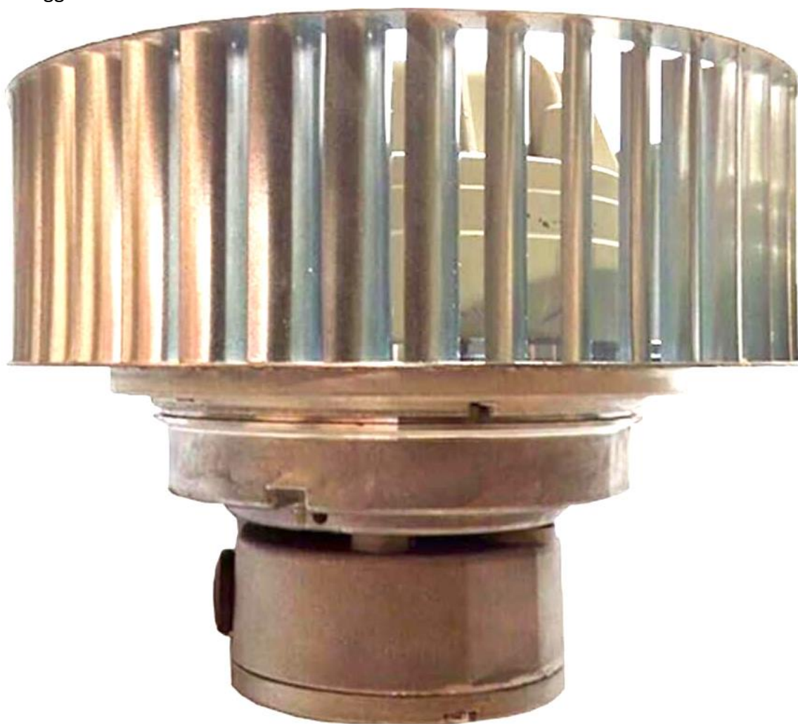
Ziehl-Abegg RE22P-2DK.3F.5R
