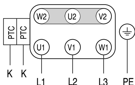
(Y) Schaltung / Star connection
