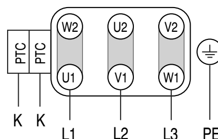
( \Delta ) Dreieckschaltung / Delta connection
