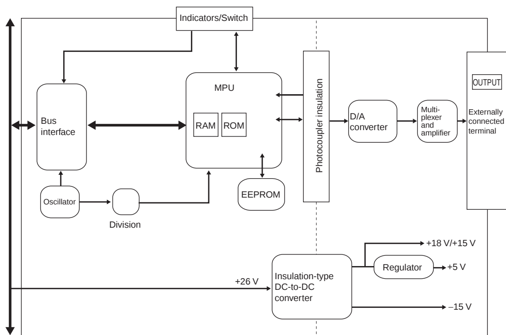
CS-series PLC
