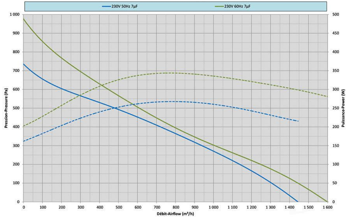
Courbes Débit/Pression-Puissance Airflow/Pressure-Power Curves E04-A5 2RRE45 280x40R (Inv)
